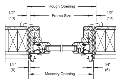
JAMB - PICTURE
