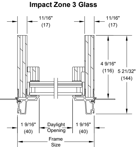
Jambs
